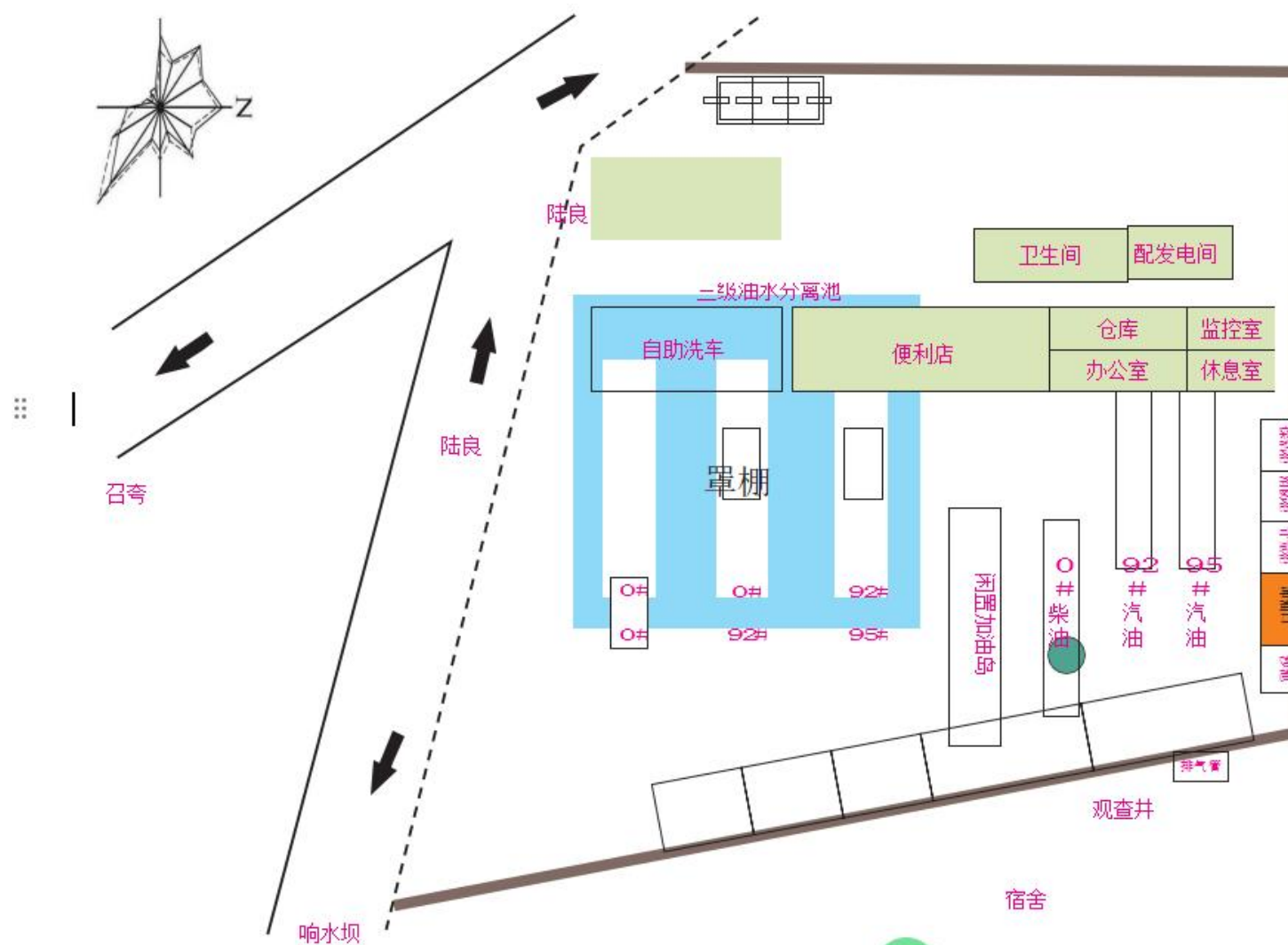
图2.4-1平面布置示意图
