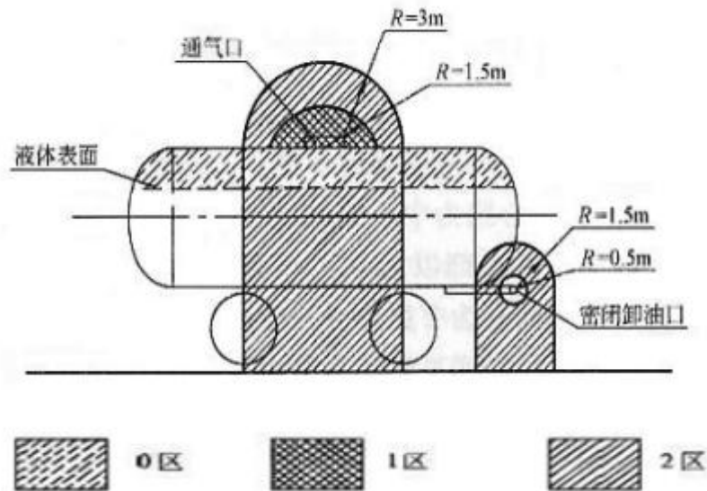
图 3.7-3 汽车油罐车和密闭卸油口爆炸危险区域划分
