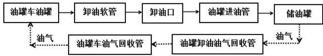
图2.5-3 汽油卸油工艺流程框图
