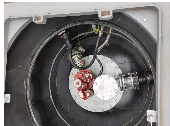
图 8 油罐操作井 B
