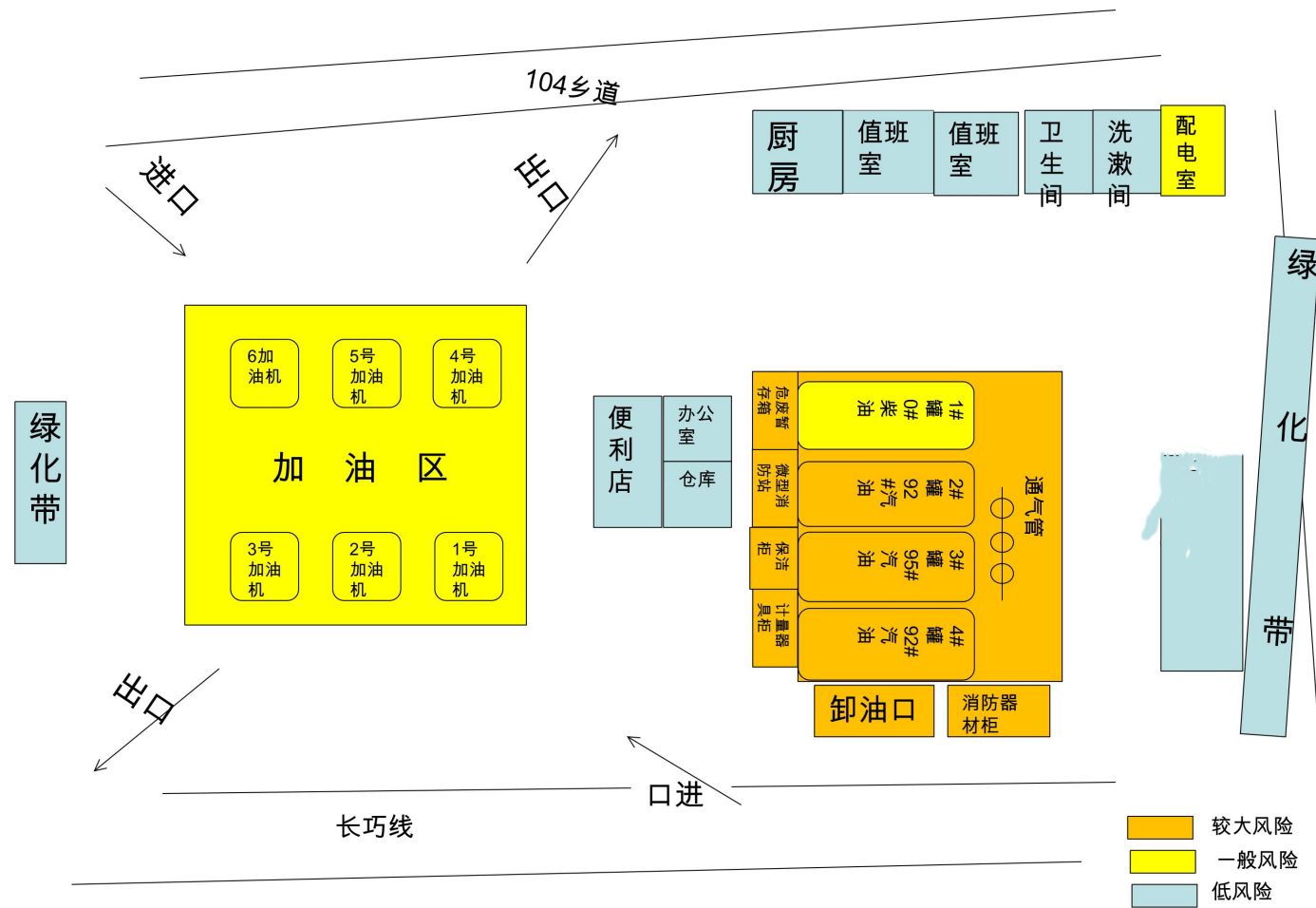
环东加油站平面布局图
