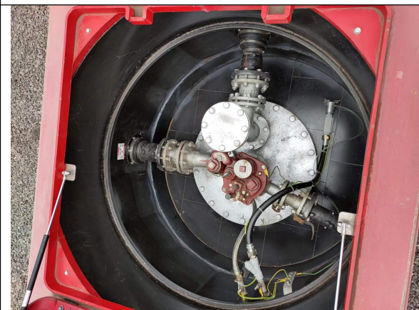
图 7 油罐操作井 A
