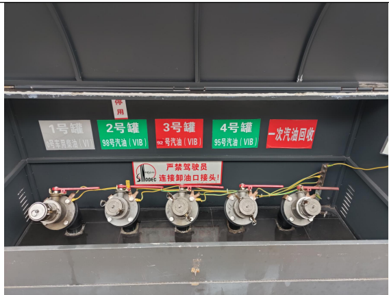
图 7 卸油口
