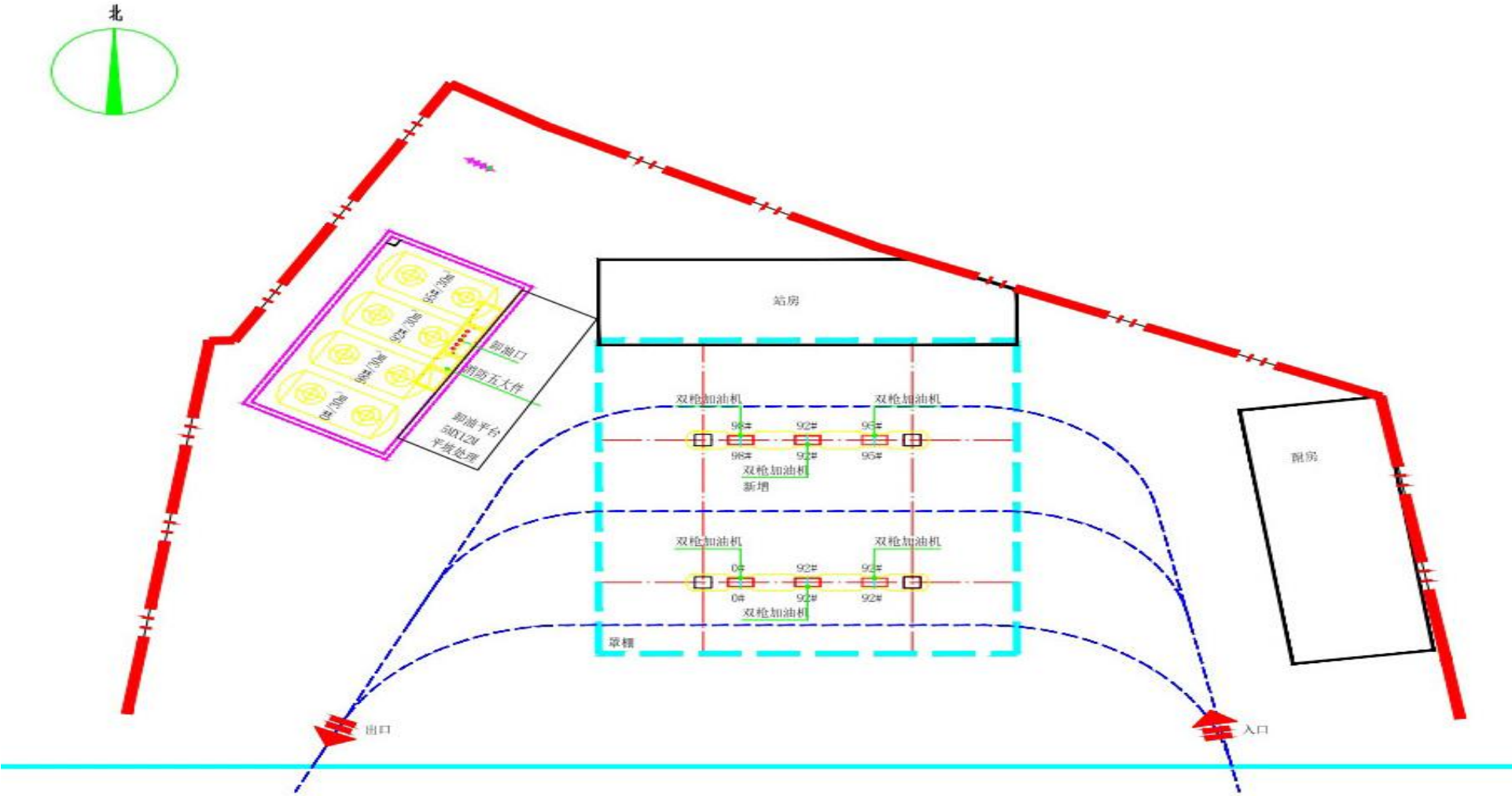
附件 19 加油站总平面布置图
