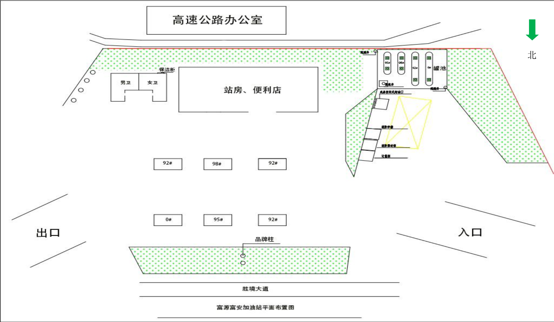
图2.3-1富安加油站总平面布置图
