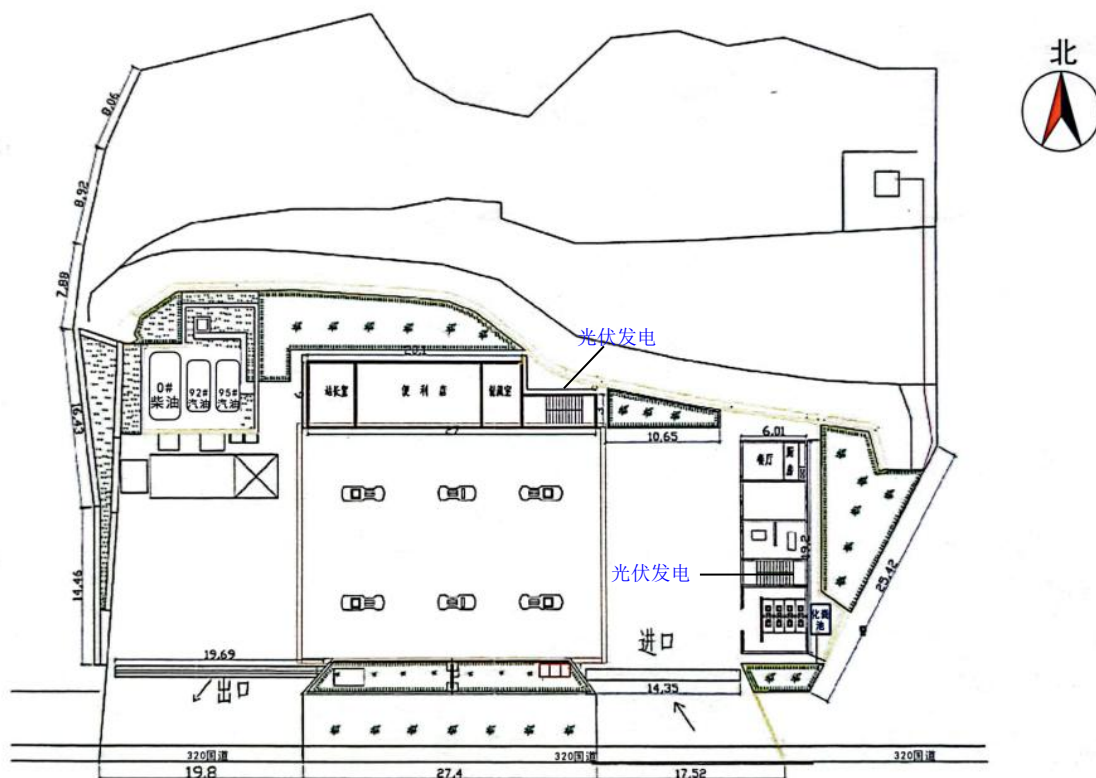
王家屯加油站平面图
