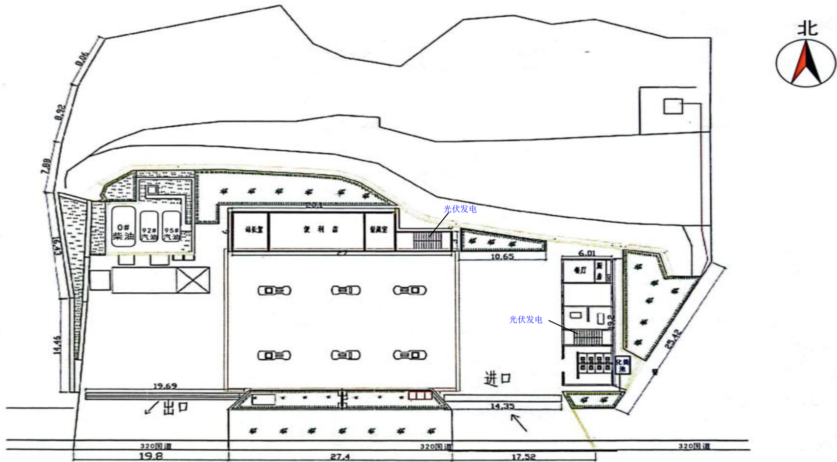
王家屯加油站平面图
