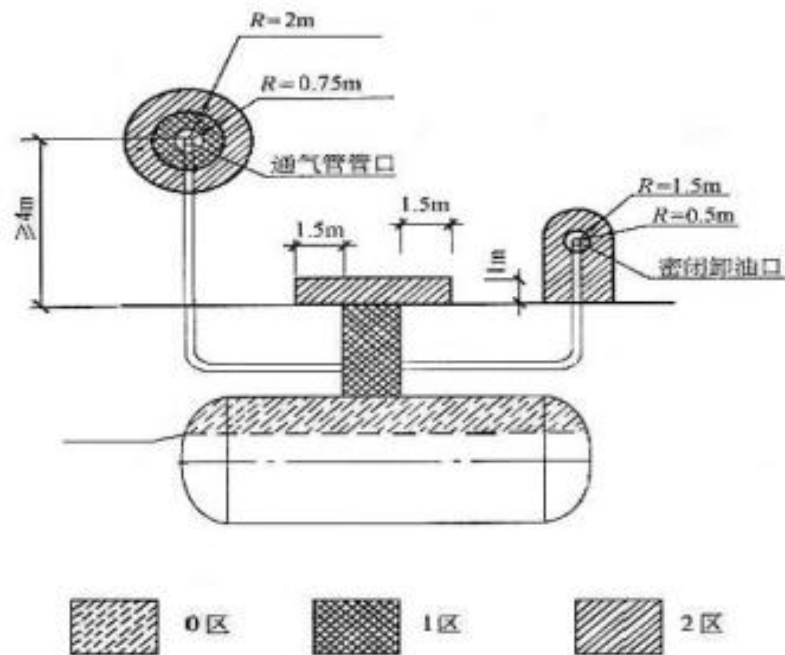
图 3.7-1 埋地油罐防爆区域划分图
