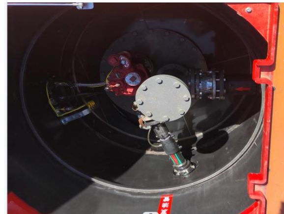
图18 操作井
