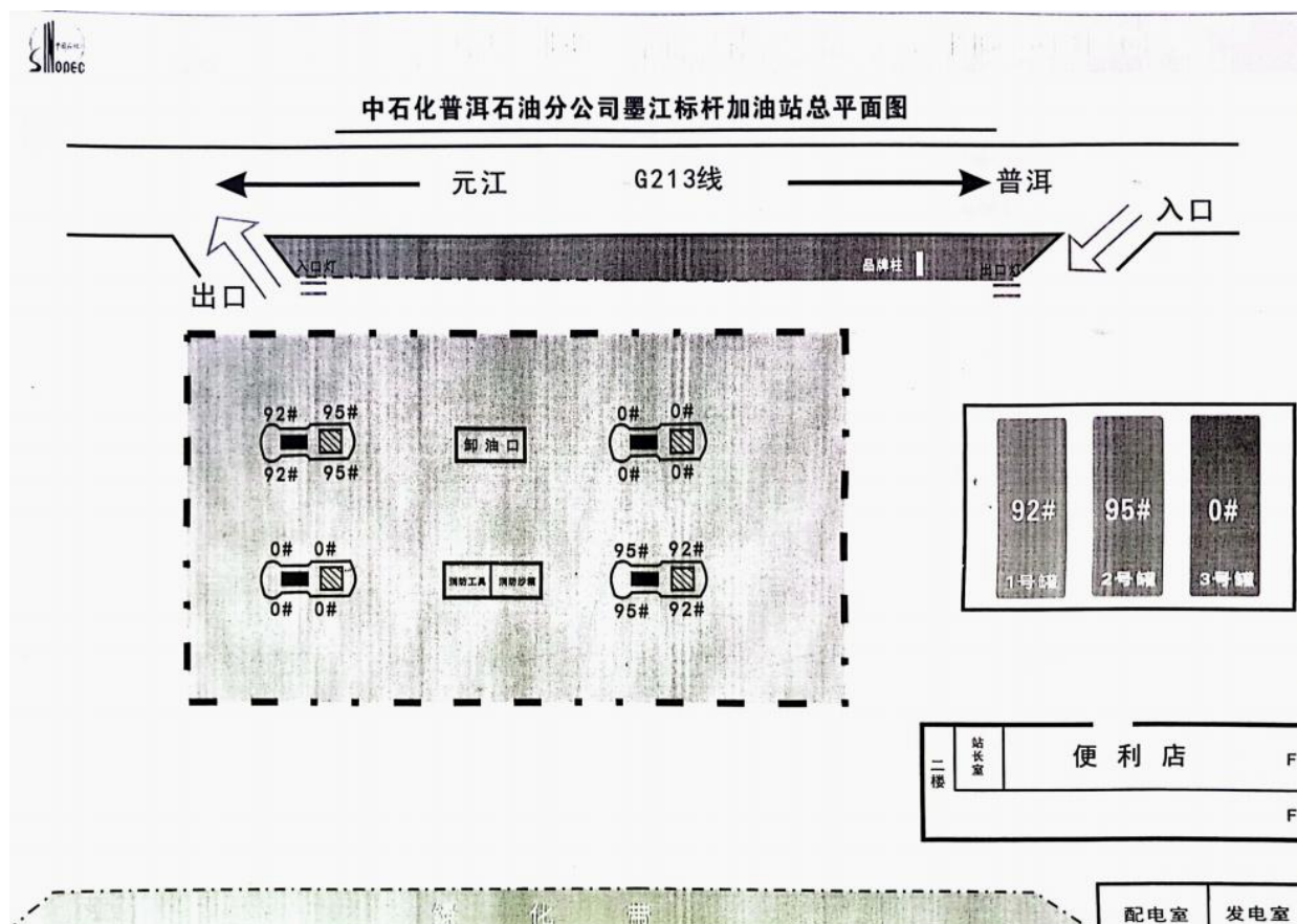
图2.3-1 总平面布置示意图
