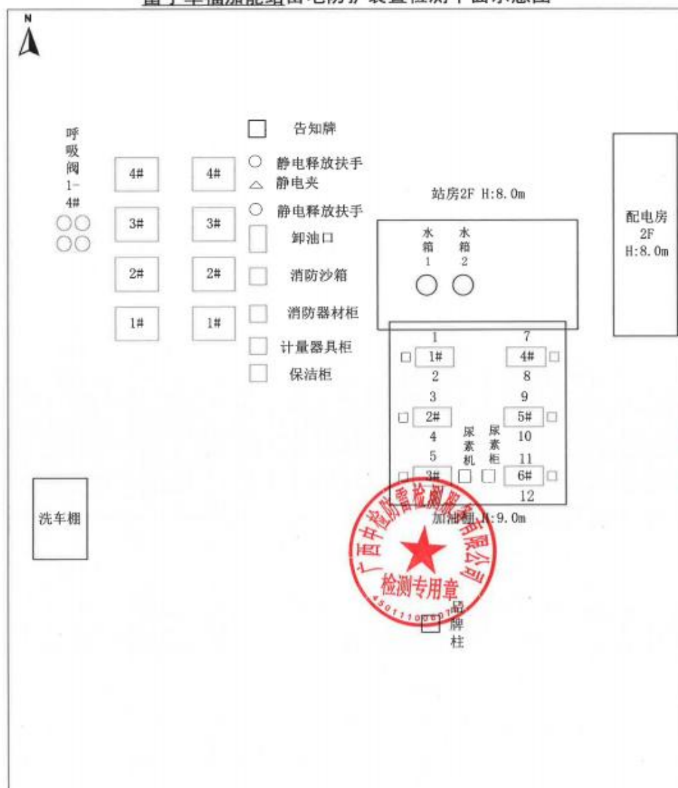
富宁幸福加能站雷电防护装置检测平面示意图
