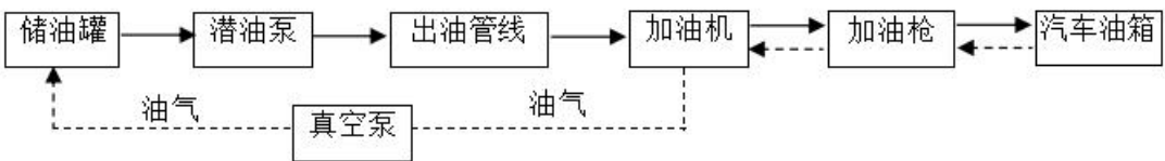
图2.4-1加油工艺流程图
