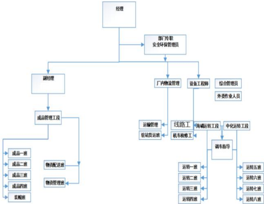
图2-14 组织架构
