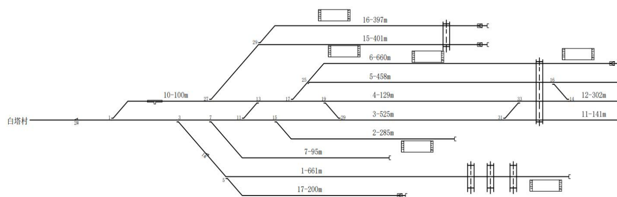
图2-1 专用线平面图
