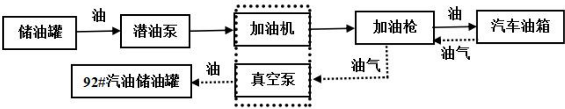
图 2-5 汽油加油工艺流程框图
