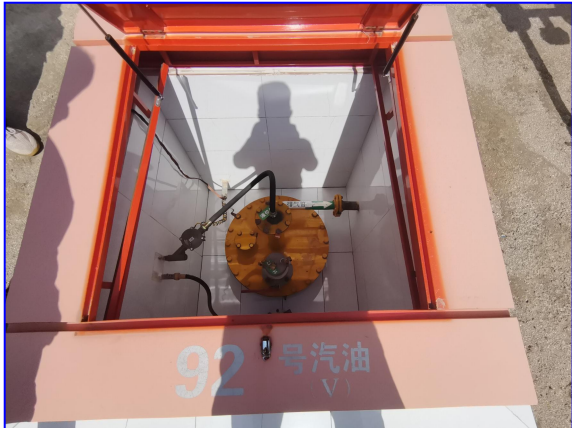
图 9 油罐操作井—92#-1
