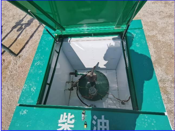
图 12 油罐操作井—0#-2
