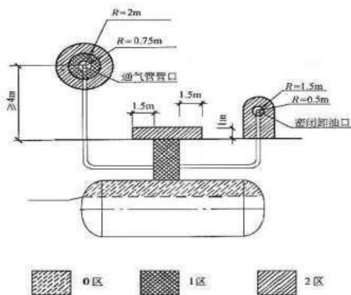
图 3-1 埋地油罐防爆区域划分图
