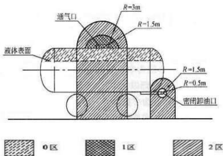
图 3-3 汽车油罐车和密闭卸油口爆炸危险区域划分
