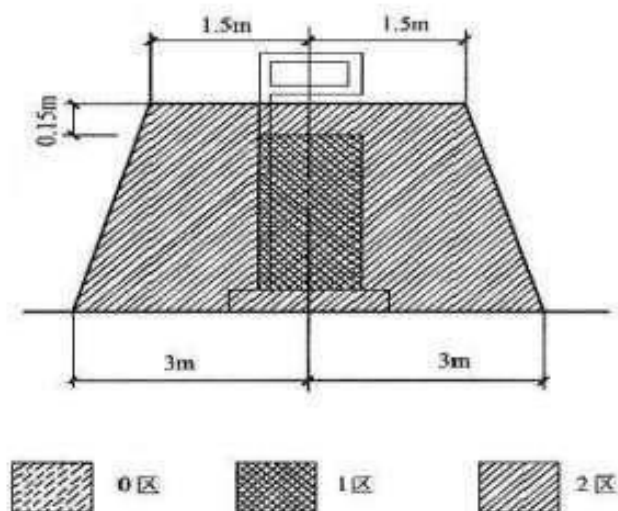
图 3-2 加油机防爆区域划分图
