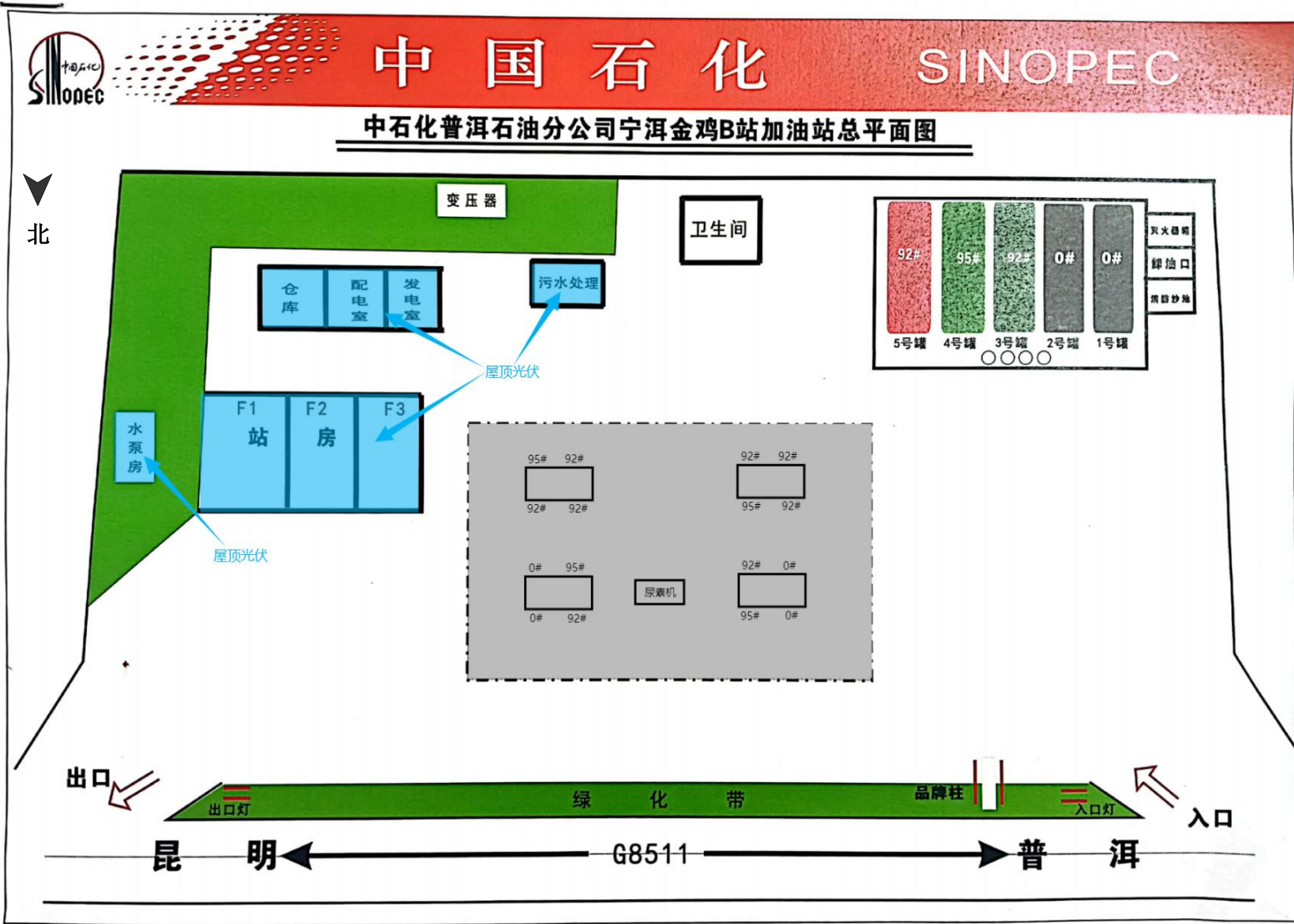
附件 16 加油站总平面布置图
