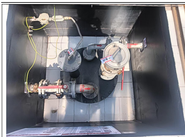
图 17 量油孔操作井
