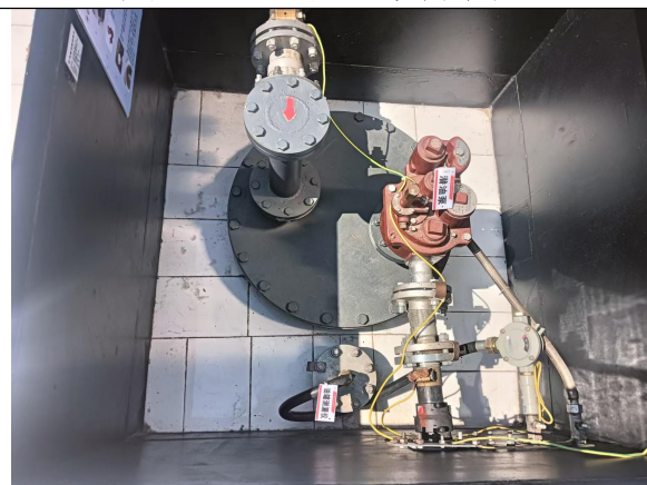
图 16 潜油泵操作井
