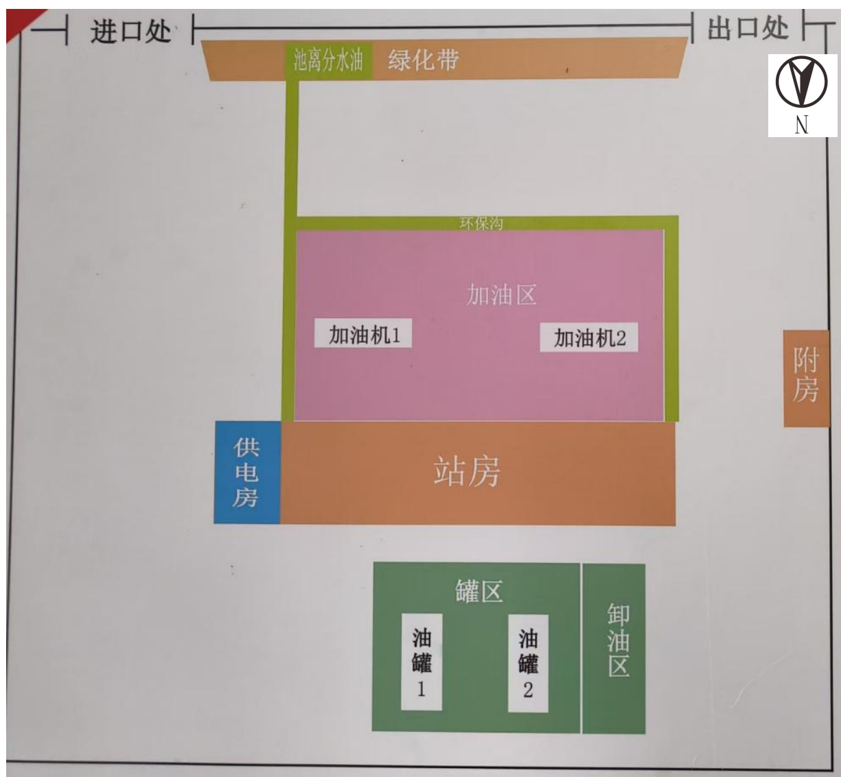
附件 14 加油站总平面布置图
